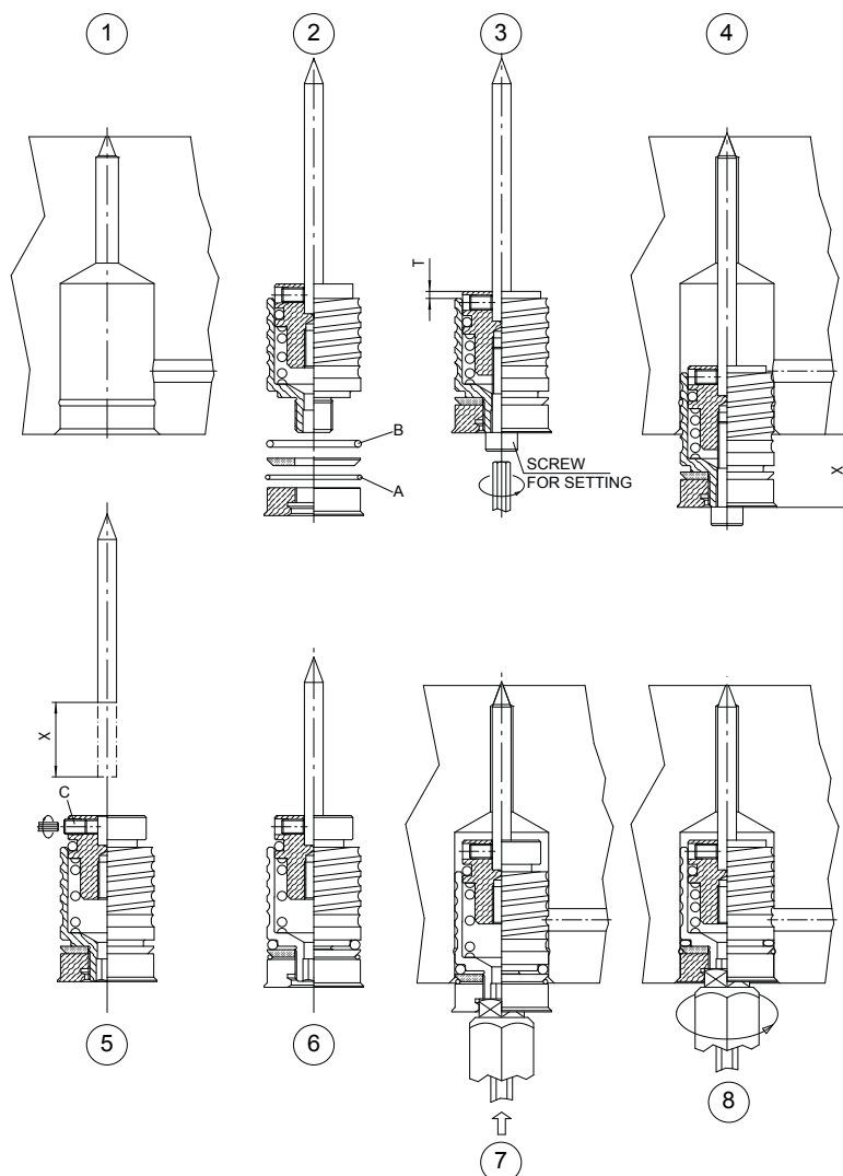
Посадочное гнездо
