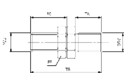
Metric Male Thread Метрическая наружная резьба
