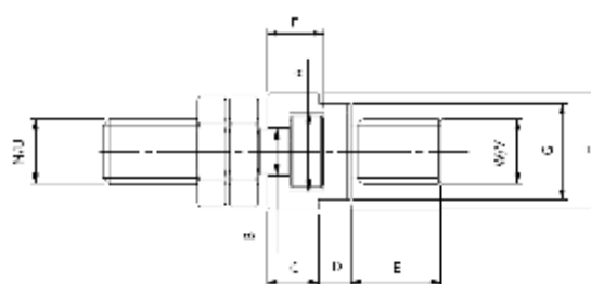
Floating Joint With Female Плавающее соединение с наружной резьбой
