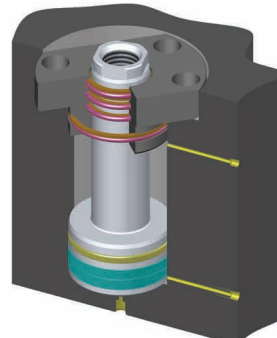
Flanged Cartridge Cartuccia flangiata
